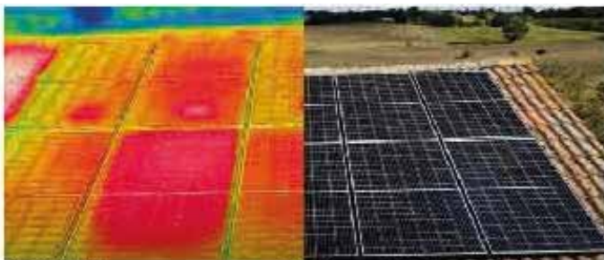
Défaillances sur cellules photovoltaïques
